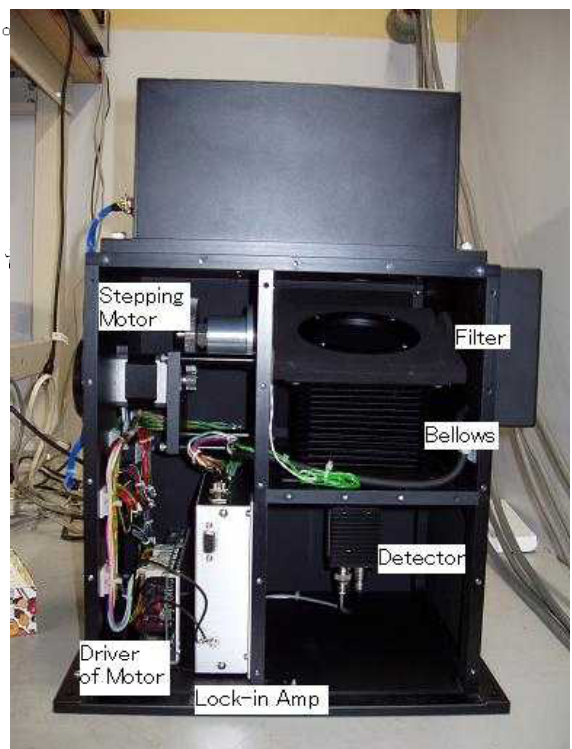
図1 Tilting Filter Potometer の構造
