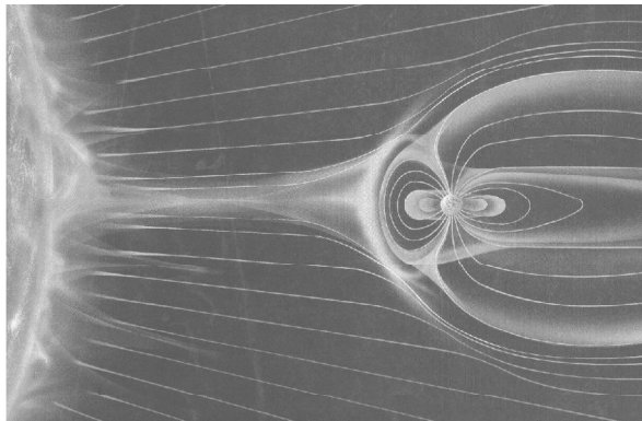
図1:地球近傍の宇宙空間プラズマの概念図 写真1:幾重にも折り重なったオーロラの例 太陽(左)から吹き出す太陽風と地球磁気圏(右)
