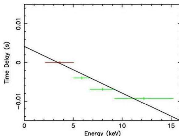
図1. ブラックホール候補星 GRS1915+105 の時間変動。変動の時間のずれをエネルギーの関数で表した。エネルギーの高い X 線ほど早く変動することを発見した。(Ohkawa, Kitamoto & Kohmura, 2005, ApJ, in press)
