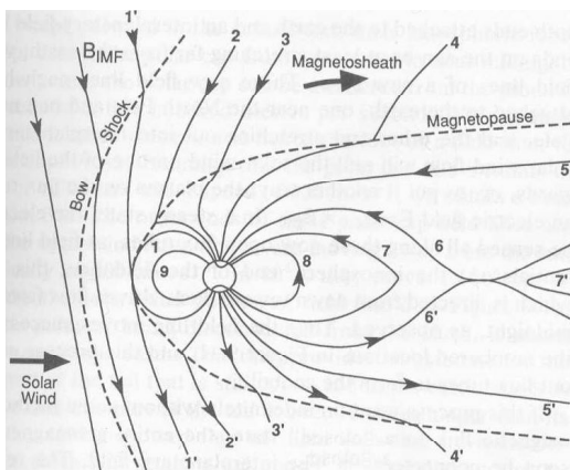
図 2:磁気圏前面(1)と尾部(6)での磁力線再結合 図 3:ISTP の科学探査人工衛星群
