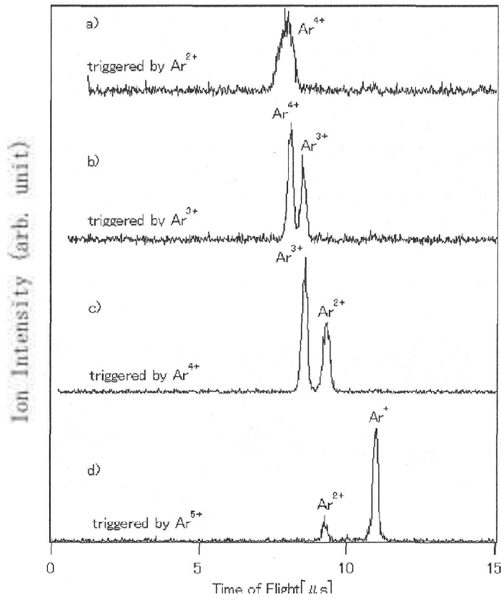
図1. \text{Ar}^{6+} イオン（入射エネルギー2.4keV）とAr原子の衝突で生成される多価イオンの同時計測スペクトル。
