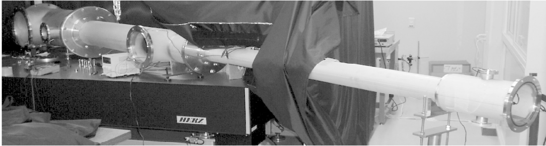
図3. Xmas 計画で進めている X 線望遠鏡の実験装置、長さ 4.5m の真空槽が望遠鏡の鏡筒である。
