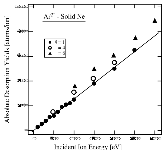
図 3: \text{Ar}^{q+} ( q = 1, 4, 6 ) 衝撃による固体 Ne からの脱離収率の入射イオンエネルギー依存性。実線は \text{Ar}^{+} に対するフィッティング直線。
