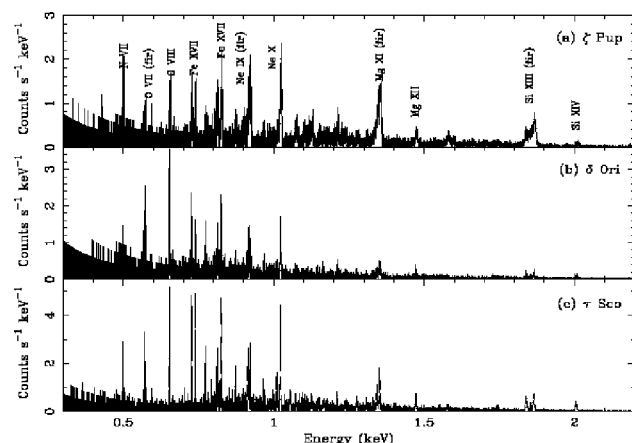
図 2. チャンドラ衛星が観測した 3 つの大質量星の X 線エネルギースペクトル。たくさんの輝線が検出されている。(Yamamoto, Kitamoto, Takano, Kohmura 2005 submitted)。
