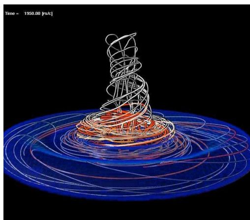
図 2 : 磁気降着円盤モデル。国立天文台のスーパーコンピュータによる数値シミュレーション[(C)Y.KATO]
