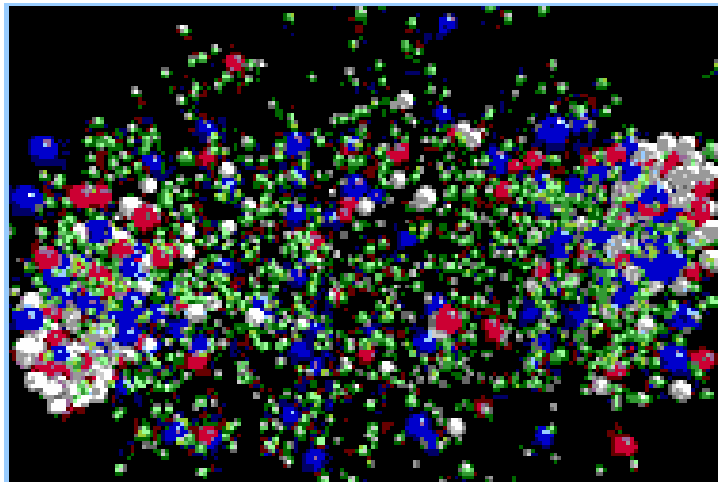
図1 : 核子あたり 100GeV の金原子核の正面衝突から生成されるおびただしい数の粒子群イメージ
