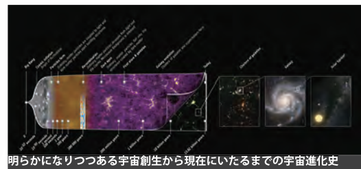
明らかになりつつある宇宙創生から現在にいたるまでの宇宙進化史
