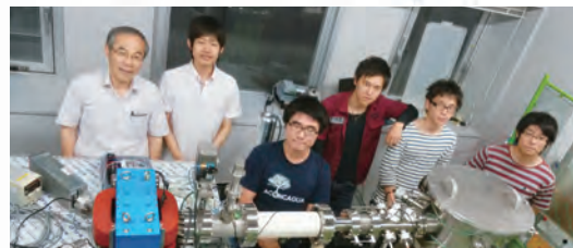
上：SCRIT 電子散乱実験初の物理結果
