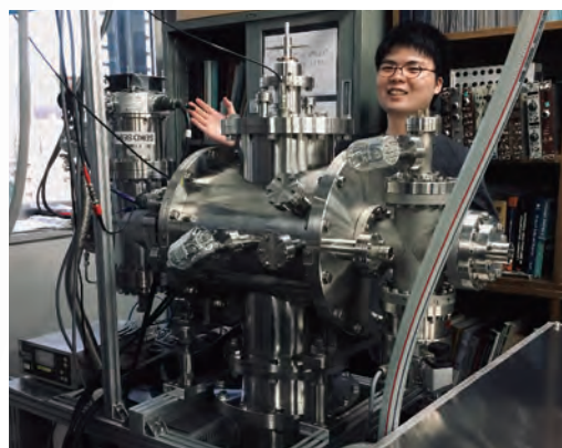
極低温・極低密度条件下における異性体と水素分子などの反応を調べるための移動度分析装置
