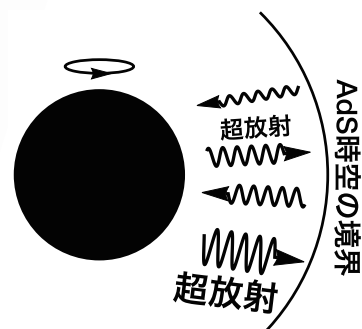
超放射不安定性の概念図：AdS時空では境界があるために超放射現象による増幅が続くことができ、不安定性が起こりうる。
